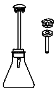
图2 砷化氢发生瓶和测砷管
