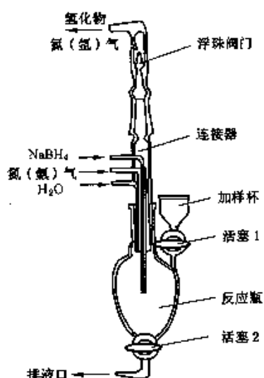
图3 反应器示意图
