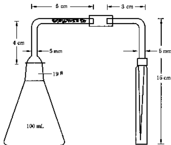
图 1 砷化氢发生瓶及吸收管
